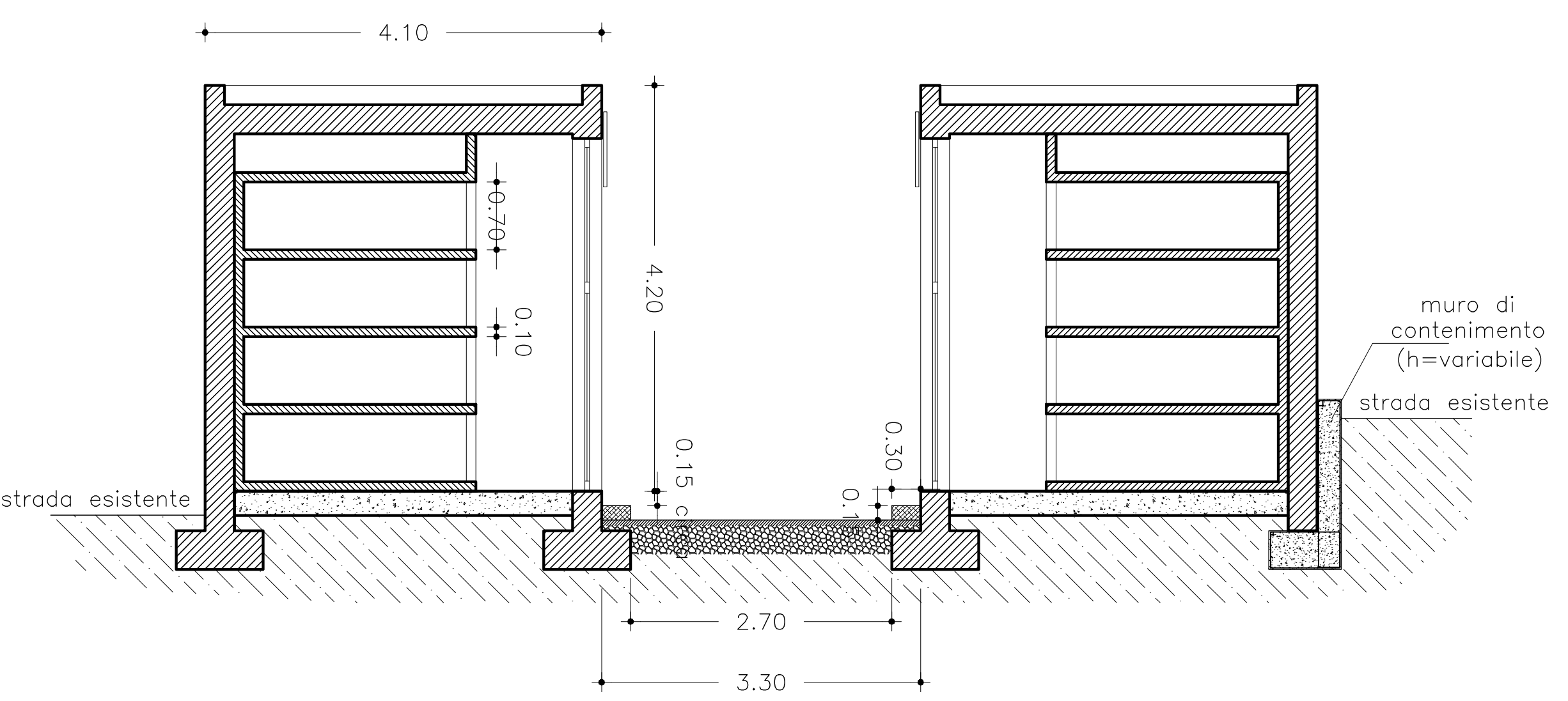
SEZIONE A-B
